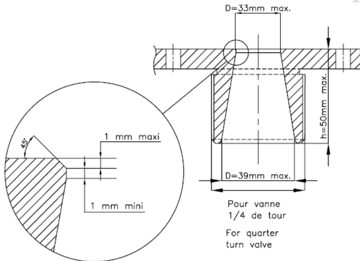
Dessin Tekening 258-3
