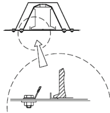
Dessin Tekening 255-11
